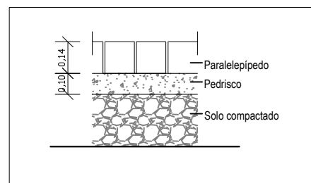
Detalhe calçamento - pedras regulares Esc: 1/25
