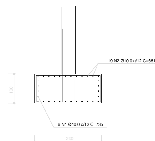
DETALHE BLOCO Corte
