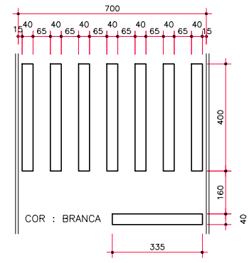
FAIXA TRAVESSIA PEDESTRES ESCALA 1:100
